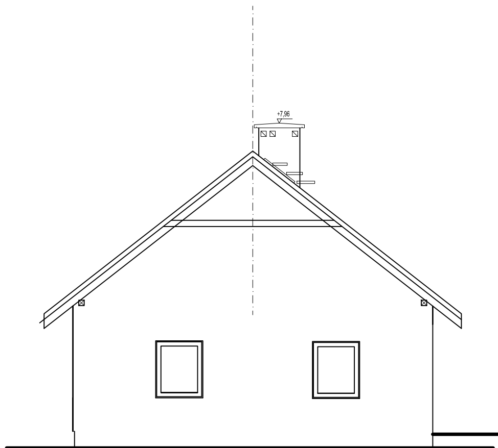
Elewacja zachodnia
